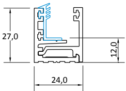
Τομή προφίλ αλουμινίου
